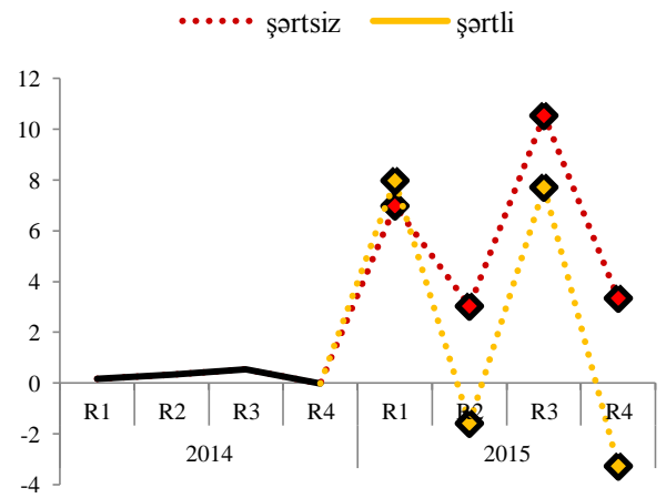
Şəkil 43. İnflyasiya
