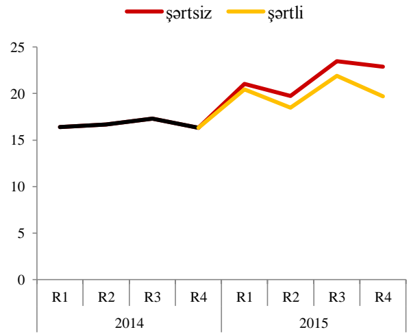
Şəkil 43. İnflyasiya
