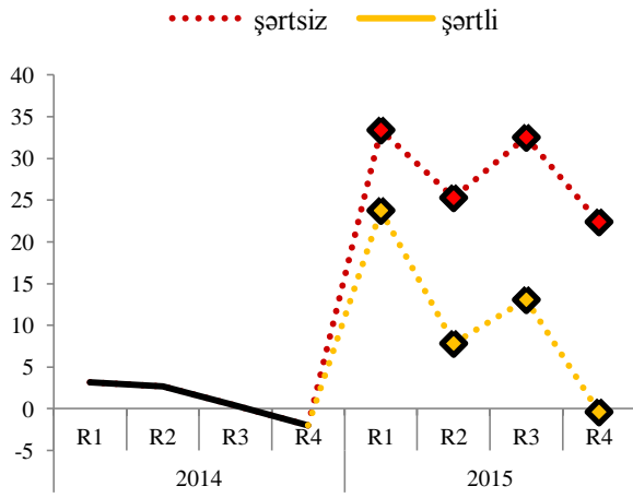
Şəkil 42. İQİ
