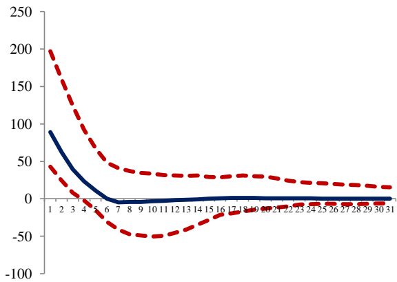
Şəkil 29. İnflyasiya
